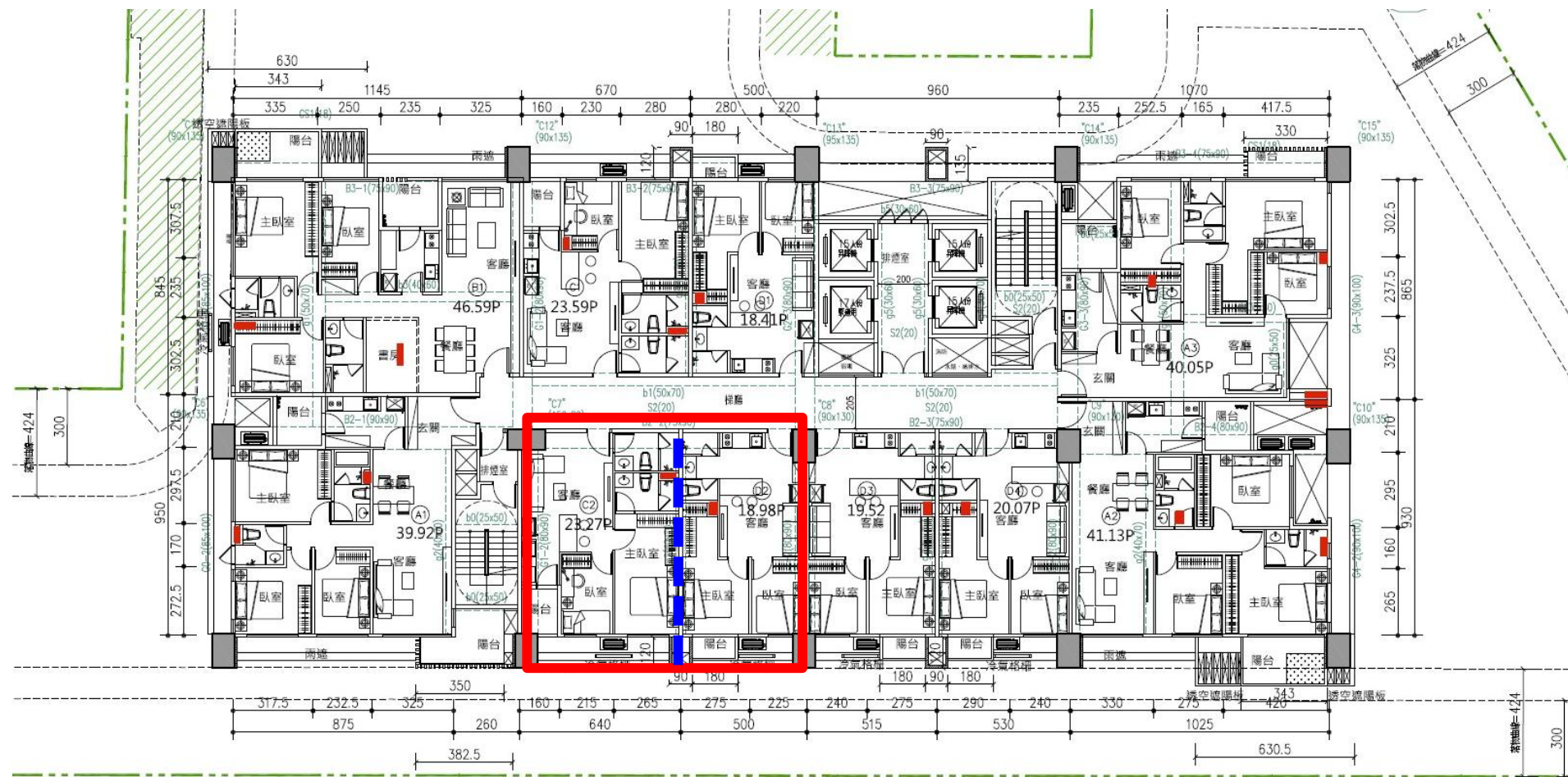
四、八、十二層平面圖 s=1/200
